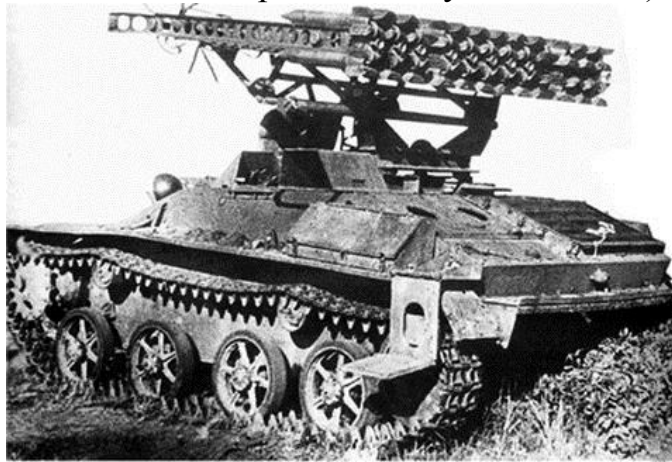
Установка для стрельбы снарядами РС-82 на танке Т-40
